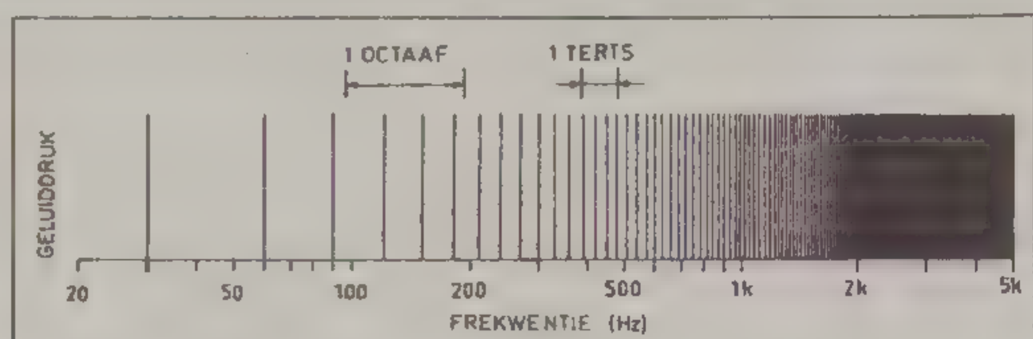
fig. 9 frekwentieresponsie van de pijp in fig. 8
